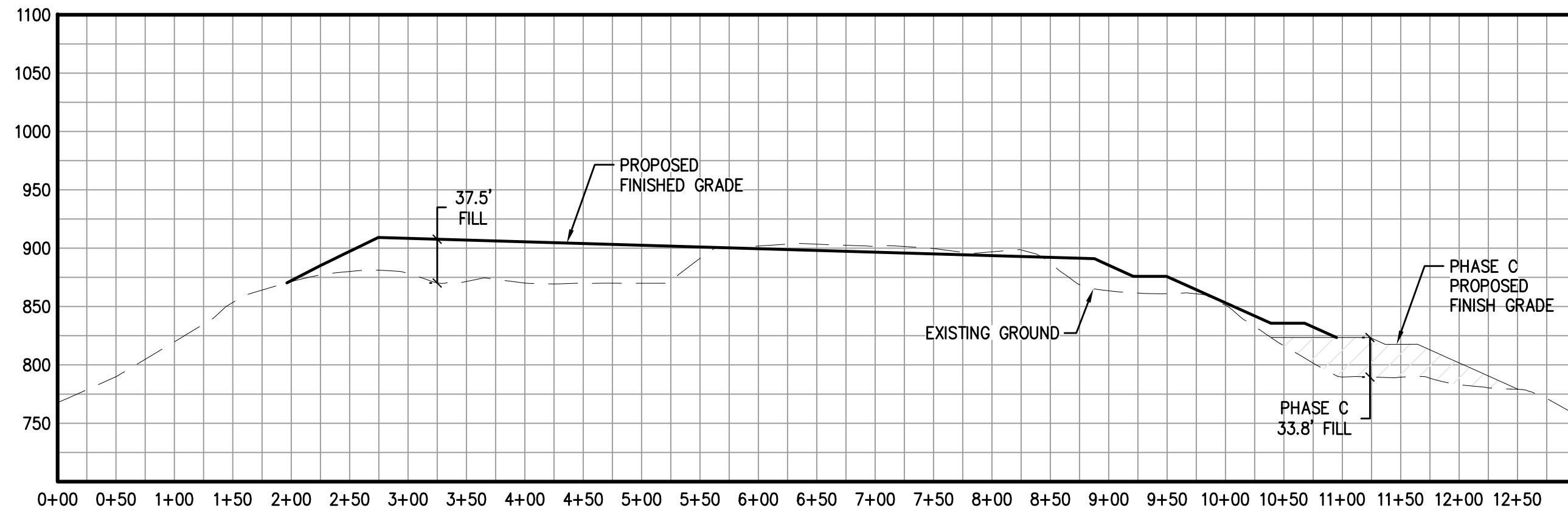
SECTION A-A SCALE: HORIZ. 1"=100' VERT. 1"=100'
