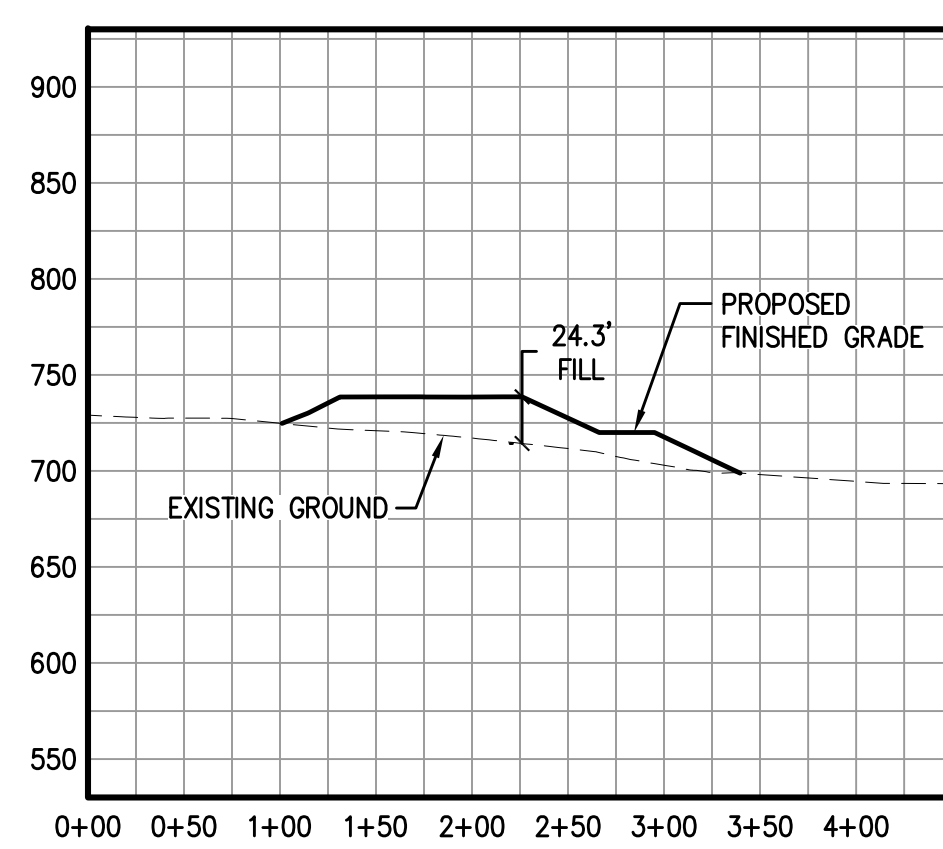
SECTION D-D SCALE: HORIZ. 1"=100' VERT. 1"=100'
