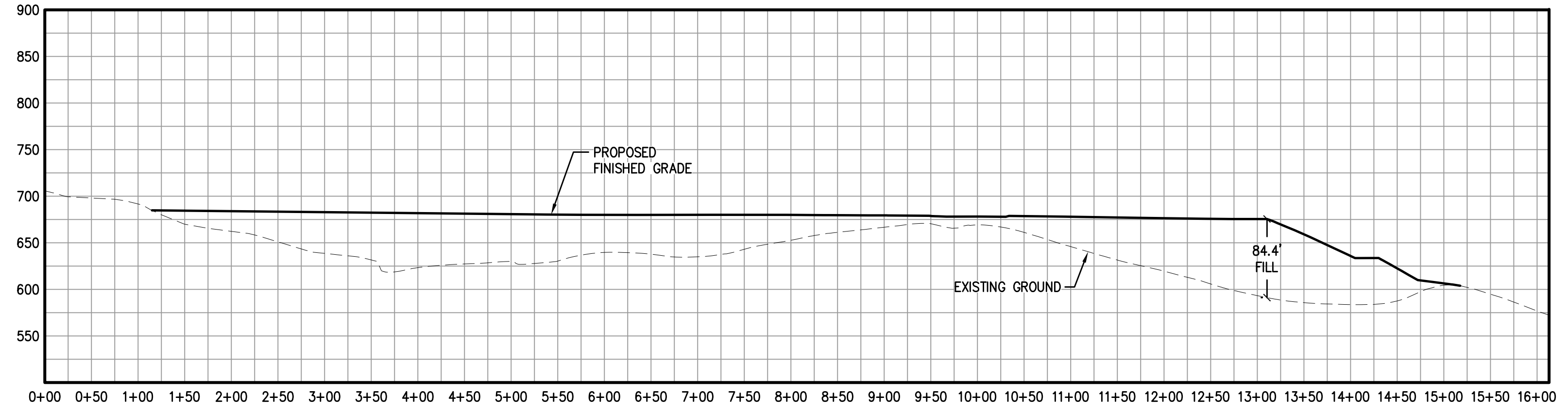
SECTION G-G SCALE: HORIZ. 1"=100' VERT. 1"=100'
